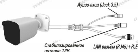
Рис. 1 Схема подключения
